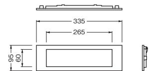
切欠図
