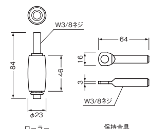
ローラー
