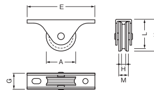
寸法表 (mm)
