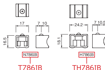
納まり図
