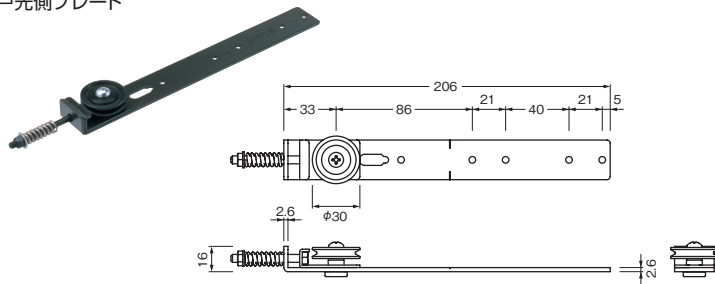
戸先側プレート
