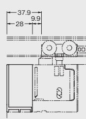
納まり図
