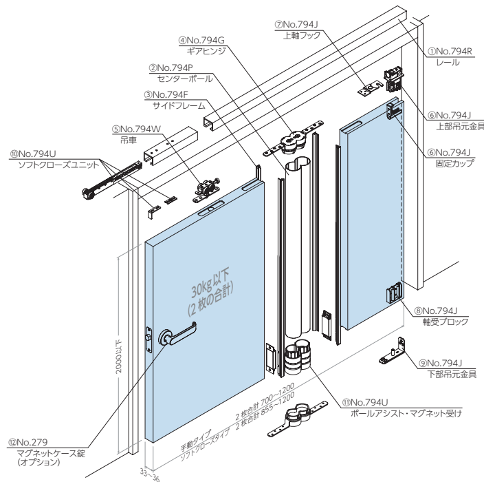
No.794SC ソフトクローズタイプ
