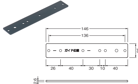
戸尻側平プレート
