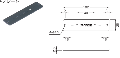
戸先側平プレート
