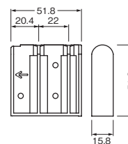
固定カップ
