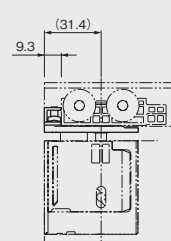
納まり図
