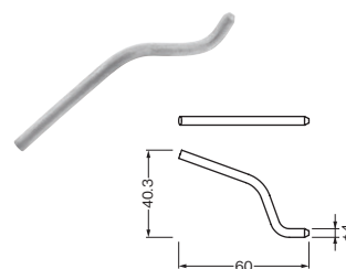
納まり図
