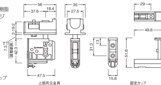
上部吊元金具
