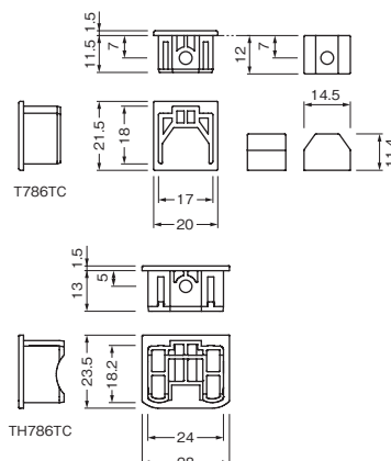
納まり図
