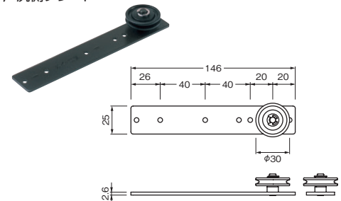
戸尻側プレート
