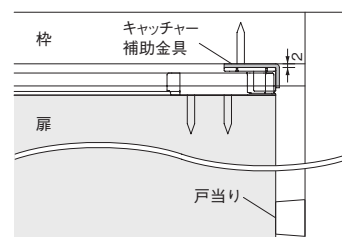
No.790-1 遮光板部品セット(別売)
