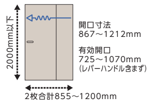
ドアの軌道図
