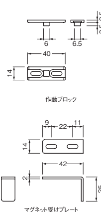
マグネット受けプレート
