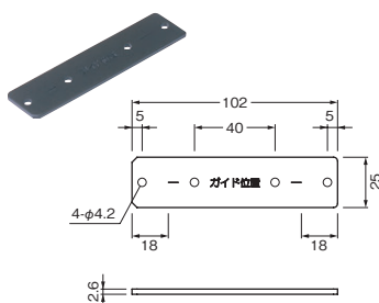
戸先側平プレート
