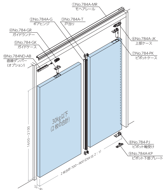
No.784A 木製ドアタイプ
