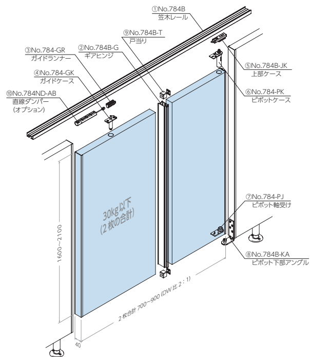
No.784B トイレブースタイプ
