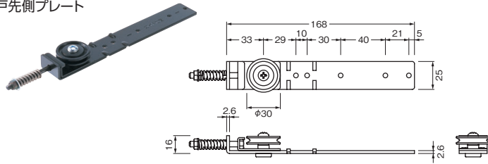
戸尻側プレート
