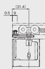
納まり図
