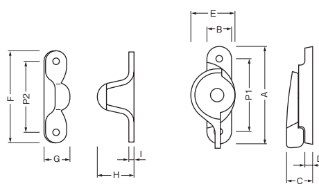
寸法表 (mm)
