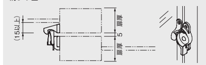
納まり図
