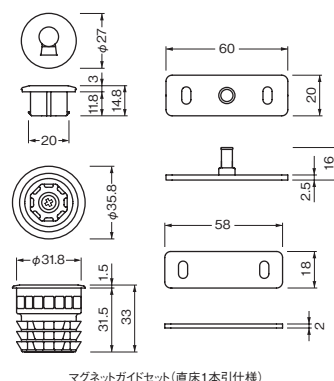
マグネットガイドセット (直床1本引仕様)
