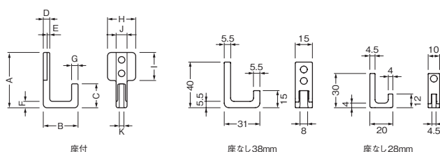
寸法表 (mm)
