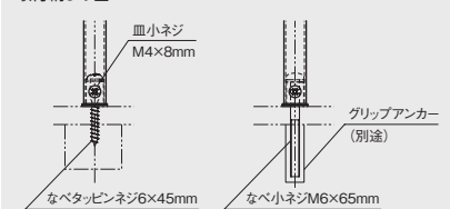
取付納まり図
