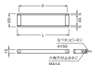
寸法表 (mm)
