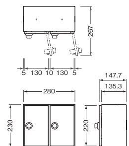
図は右勝手
