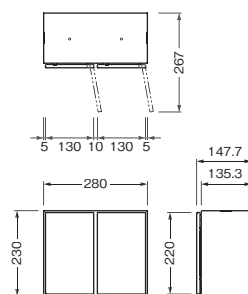
図は右勝手
