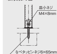
取付納まり図
