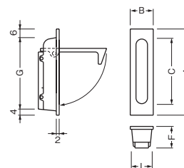
寸法表 (mm)
