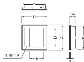
寸法表 (mm)
